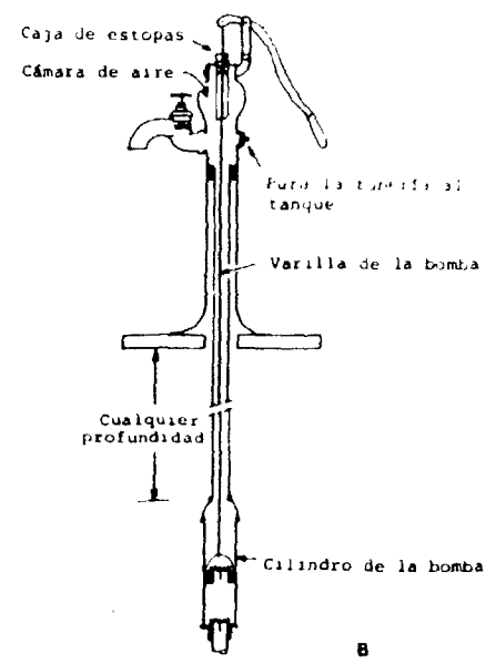
BOMBAS IMPELENTES
