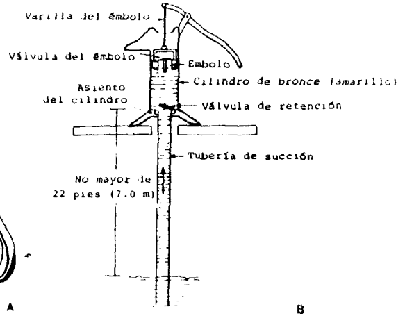
TIPICA BOMBA ASPIRANTE PARA POZO SUPERFICIAL
