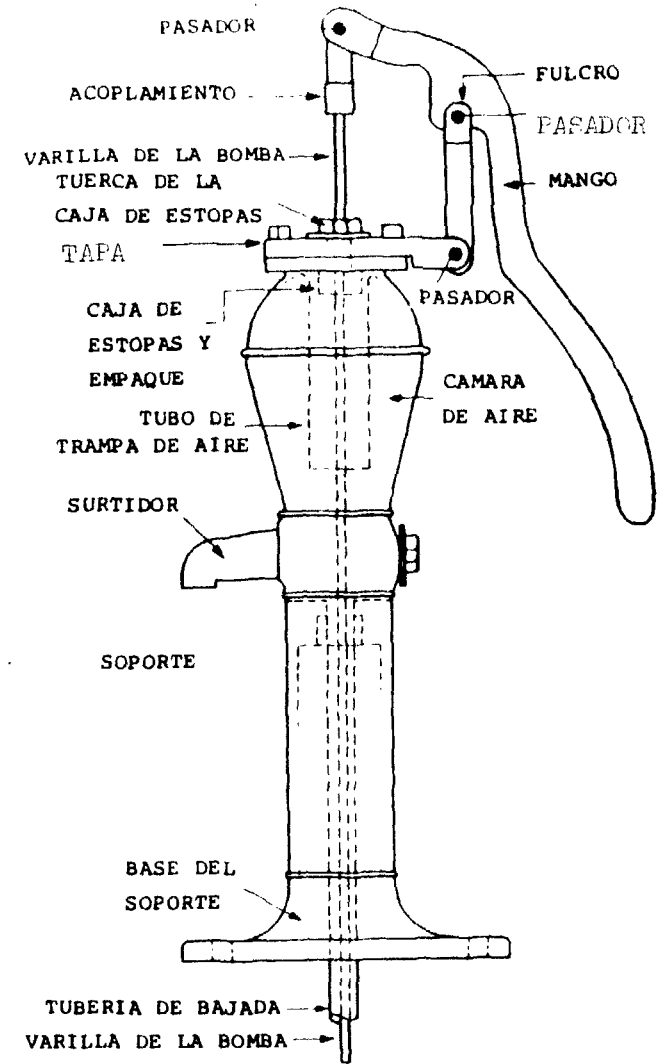
BOMBA DE MANO CON CAJA DE ESTOPAS Y VARILLA GUIADA QUE PUEDE USARSE COMO BOMBA IMPELENTE
