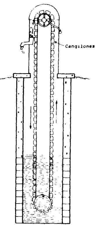
NORIA DE CANGILONES
