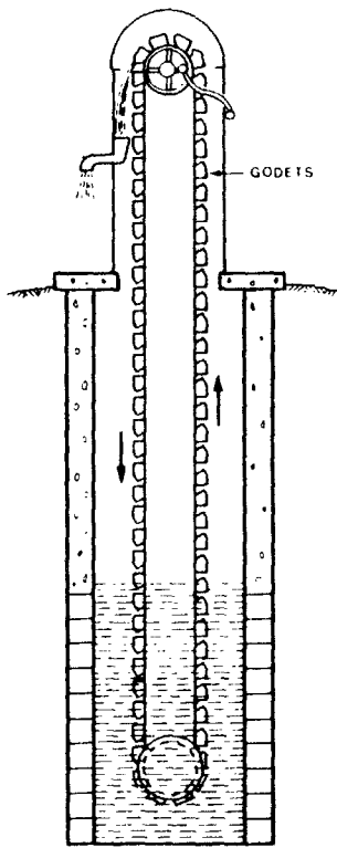
POMPE A GODETS
